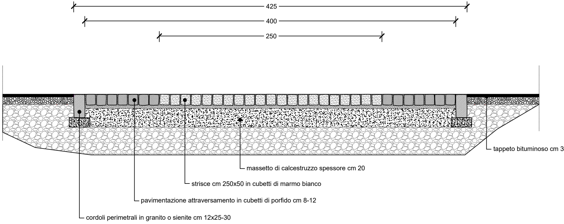
sezione tipo attraversamenti pedonali 1:25
